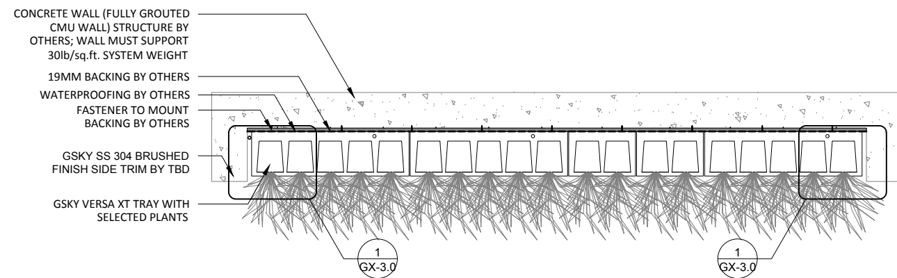
2 PLAN SCALE: 1:30
