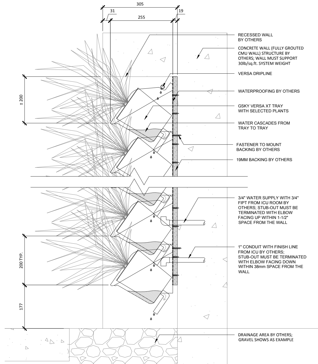
2 SECTION DETAIL SCALE: 1:8
