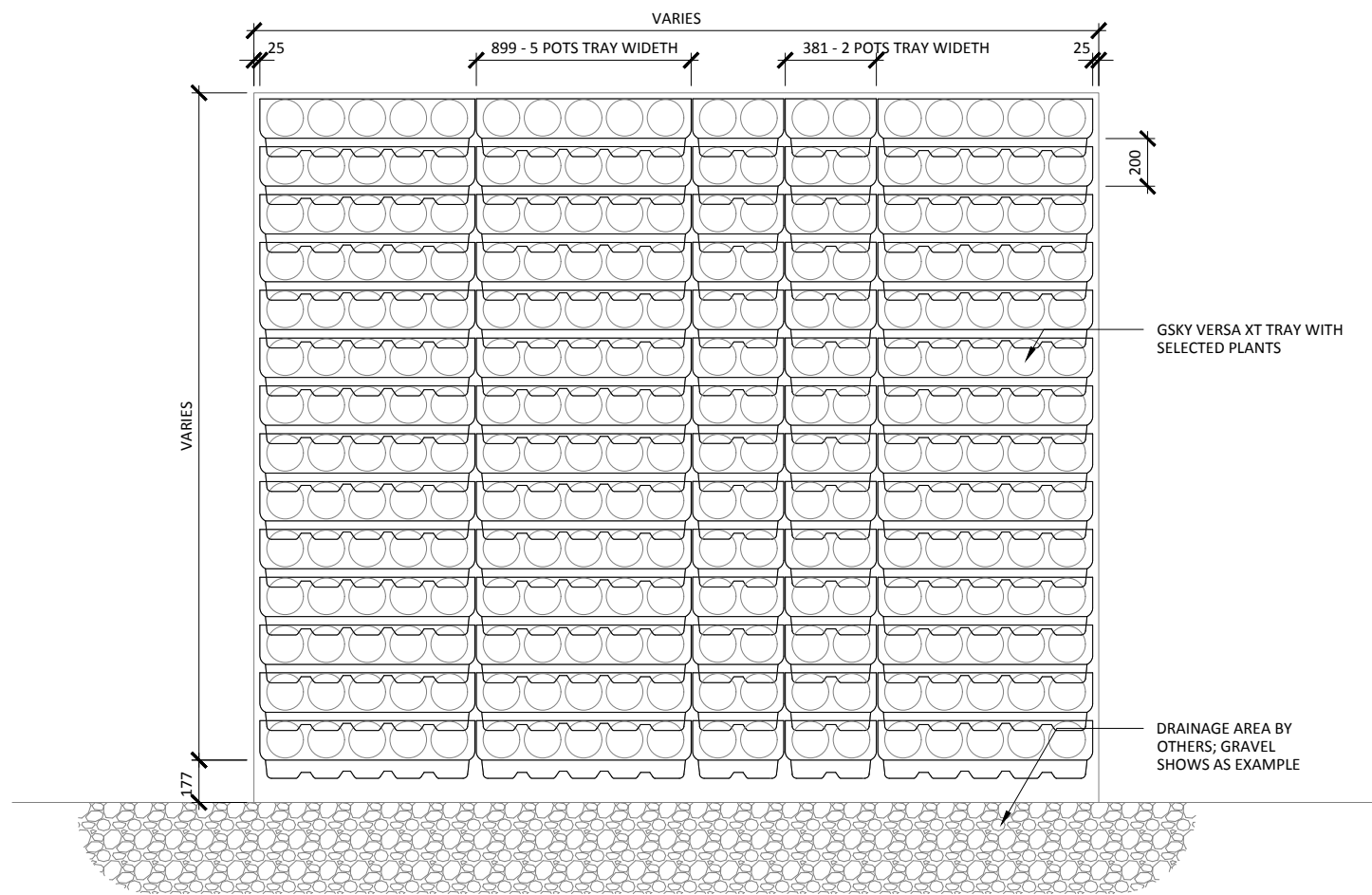
1 ELEVATION SCALE: 1:30
