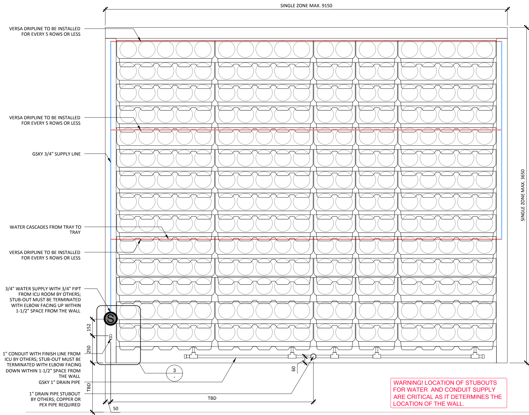
1 ELEVATION SCALE: 1:20
