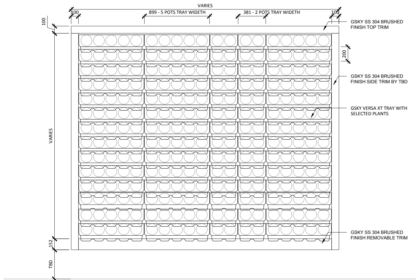
1 ELEVATION SCALE: 1:30
