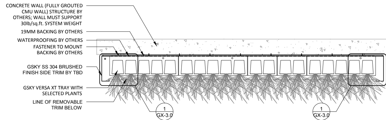
2 PLAN SCALE: 1:30
