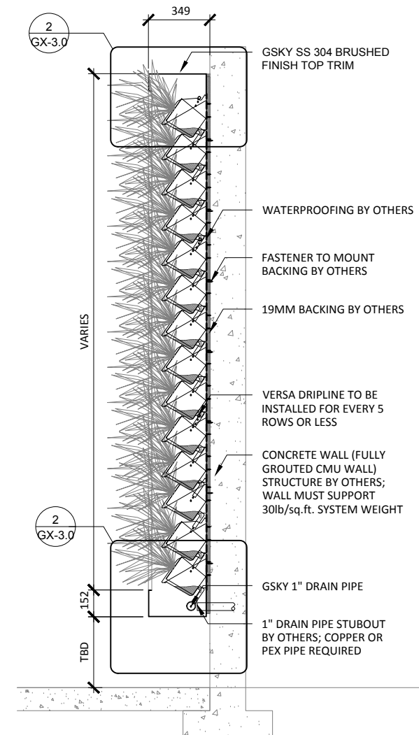
3 SECTION SCALE: 1:30
